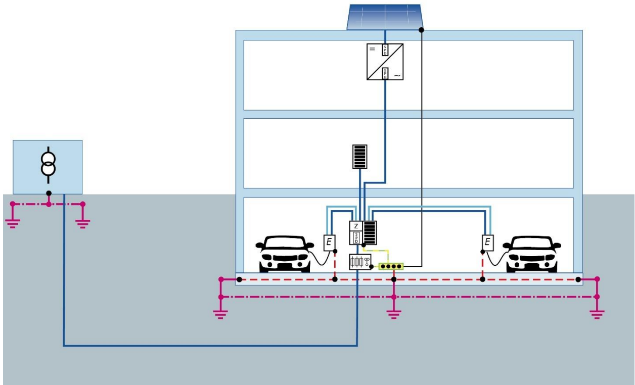
Abbildung 3: Gebäude, Kundenanlage mit Ladeeinrichtung und Erzeugungsanlage
